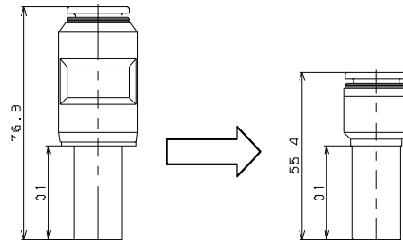
< PGJ16-12 外観寸法図 >
