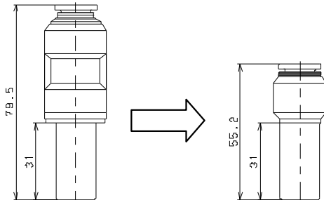
< PGJ16-10 外観寸法図 >
